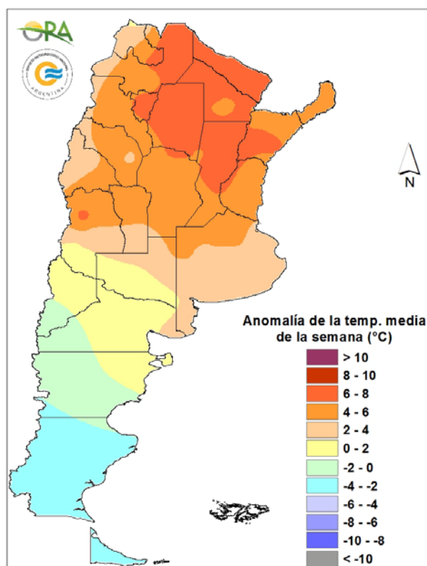
Anomalía de la temperatura media de la semana del 18/09/2024 al 24/09/2024
