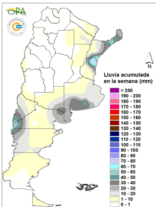
Precipitaciones acumuladas en la semana del 18/09/2024 al 24/09/2024
